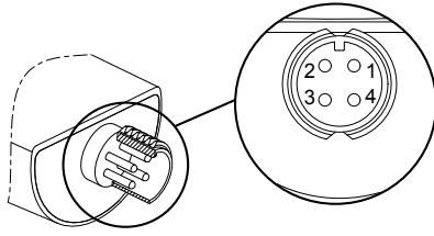
Abb. 4 Elektrische Anschlüsse
