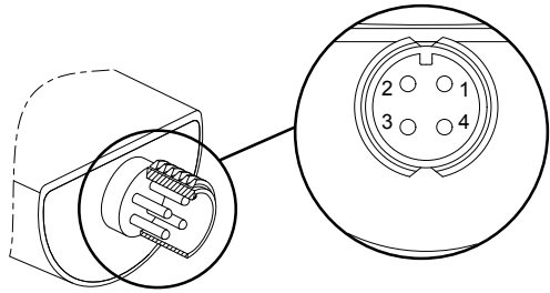
Abb. 72 Elektrische Anschlüsse
