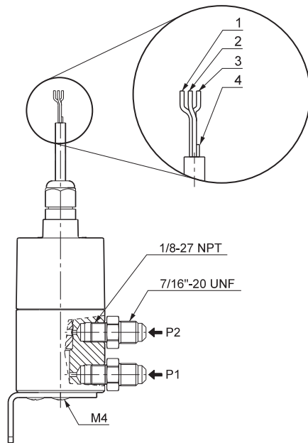
Abb. 46 Elektrische Anschlüsse
